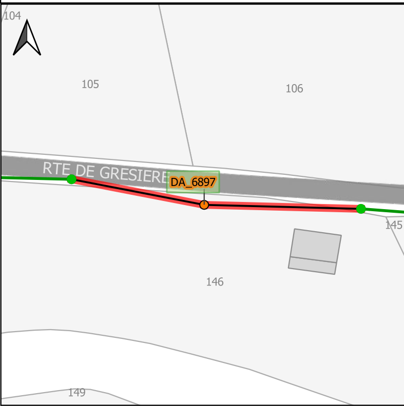
Carte d'implantation 1:1000
